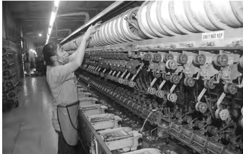
Cơ sở chế biến tơ tằm tại Lâm Hà.
